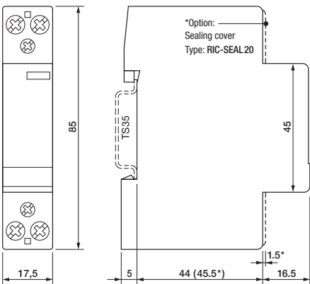
fig. 3. Abmessungen (mm)
