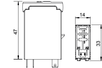
fig. 3. Dimensions (mm)
