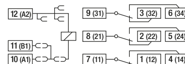
fig. 1. Wiring diagram
