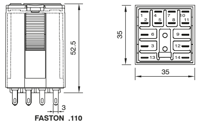
fig. 4. Dimensions (mm)
