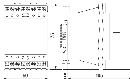
fig. 3. Dimensions (mm)
