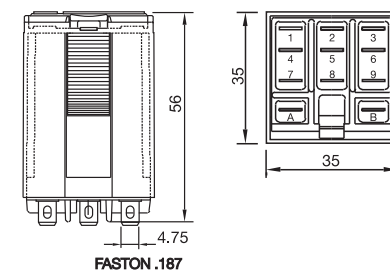
fig. 4. Dimensions (mm)
