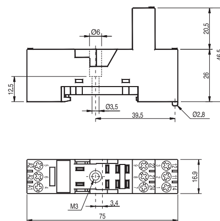
fig. 4. Dimensions (mm)
