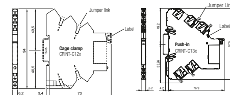
fig. 4. Dimensions (mm)
