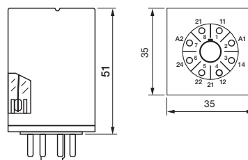
fig. 4. Dimensions (mm)
