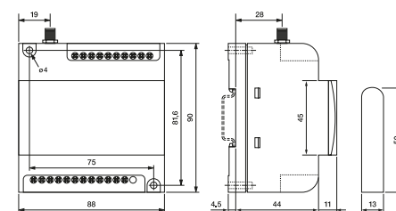
fig. 3. Dimensions (mm)
