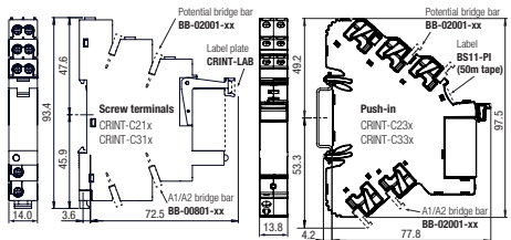
fig. 4. Dimensions (mm)
