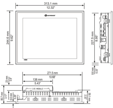
fig. 1. Dimensions (mm)
