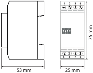
fig. 1. Dimensions (mm)
