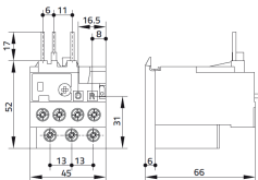
fig. 3. Dimensions (mm)
