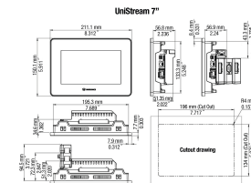
fig. 1. Abmessungen (mm)
