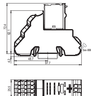
fig. 4. Abmessungen (mm)
