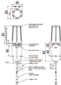
fig. 1. Dimensions (mm)
