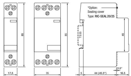
fig. 3. Dimensions (mm)
