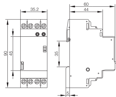
fig. 3. Dimensions (mm)
