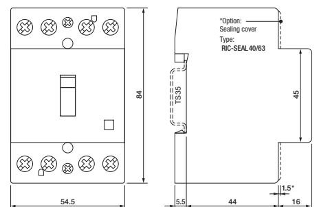
fig. 3. Dimensions (mm)
