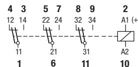
fig. 1. Wiring diagram
