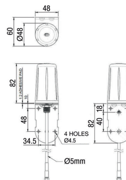
fig. 1. Dimensions (mm)
