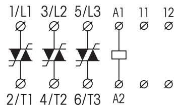
fig. 1. Wiring diagram
