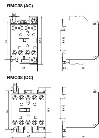
fig. 3. Dimensions (mm)
