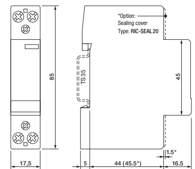
fig. 3. Dimensions (mm)
