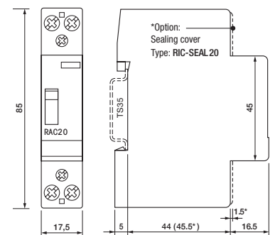
fig. 3. Dimensions (mm)
