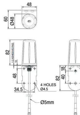
fig. 1. Abmessungen (mm)
