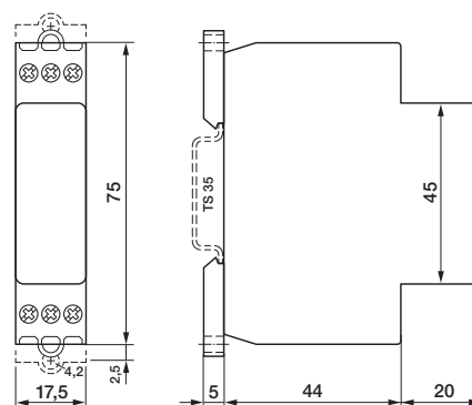
fig. 4. Dimensions (mm)
