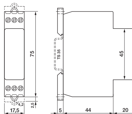
fig. 4. Dimensions (mm)
