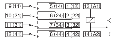
fig. 1. Verdrahtungsdiagramm
