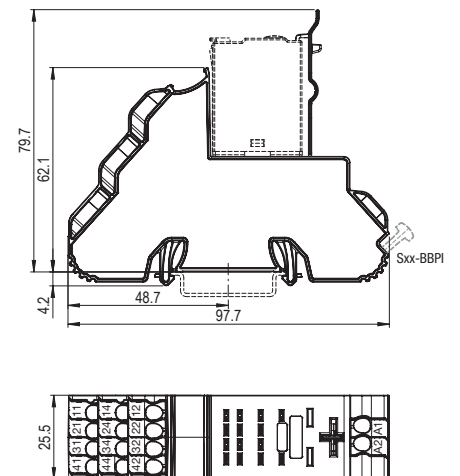
fig. 2. Abmessungen (mm)
