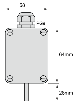
fig. 1. Dimension (mm)
