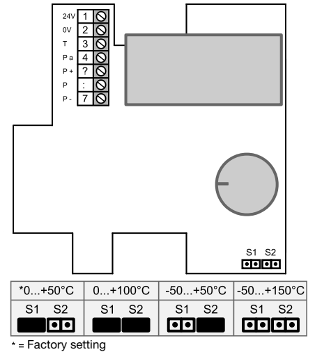
fig. 1. Wiring diagram
