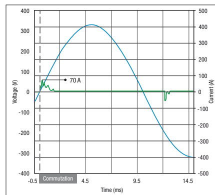
Schalten kapazitiver Verbraucher mit dem CHI14 – Einschaltstrom beträgt ca. 3.5 A pro Vorschaltgerät.
