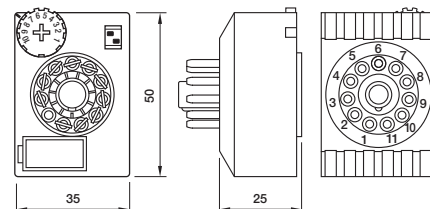
fig. 2. Abmessungen (mm)
