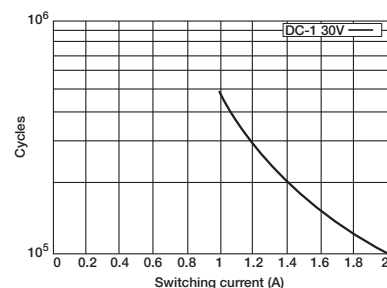
fig. 3. Gleichstrom-Grenzlastkurve
