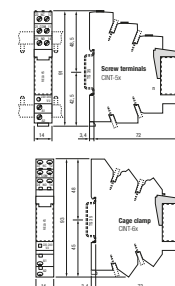
fig. 4. Abmessungen (mm)
