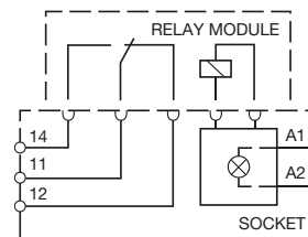
fig. 2. Wechselstrom-Schaltzyklen
