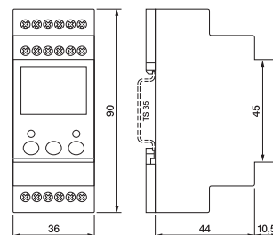
fig. 4. Abmessungen (mm)
