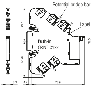
fig. 4. Abmessungen (mm)
