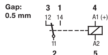
fig. 2. Wechselstrom-Schaltzyklen
