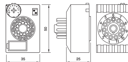
fig. 2. Abmessungen (mm)
