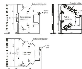
fig. 3. Abmessungen (mm)
