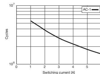
fig. 3. Gleichstrom-Grenzlastkurve
