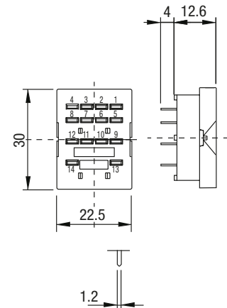
fig. 2. Abmessungen (mm)
