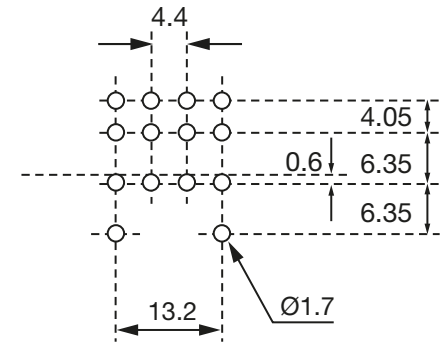
fig. 2. Abmessungen (mm)
