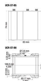
fig. 2. Abmessungen (mm)
