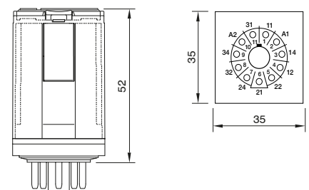
fig. 4. Abmessungen (mm)
