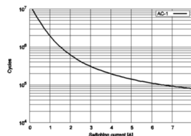
fig. 3. Gleichstrom-Grenzlastkurve
