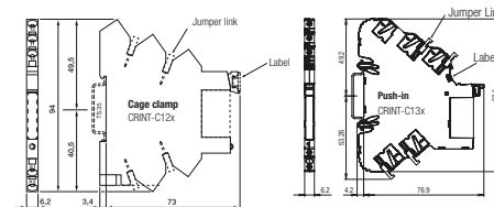
fig. 3. Abmessungen (mm)
