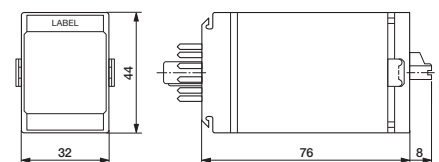
fig. 4. Dimensions (mm)
