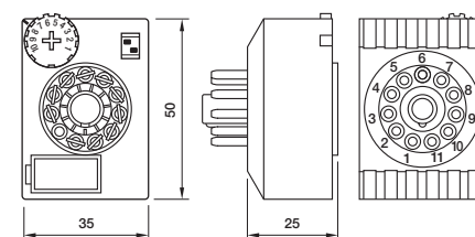
fig. 2. Abmessungen (mm)
