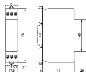
fig. 4. Abmessungen (mm)
