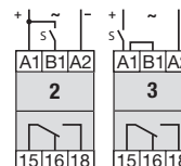
fig. 2. Wechselstrom-Schaltzyklen
