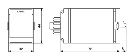
fig. 4. Dimensions (mm)
