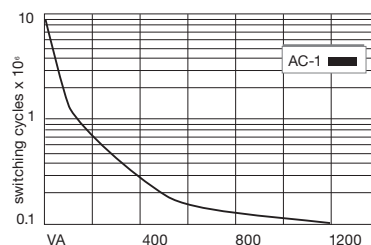
fig. 3. Gleichstrom-Grenzlastkurve
