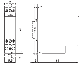
fig. 3. Abmessungen (mm)
