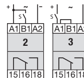
fig. 2. Wechselstrom-Schaltzyklen
